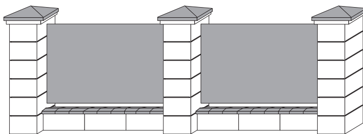
Słupek + poddasze cienkie + daszek koperta, podmurówka z daszkiem dwuspadowym
