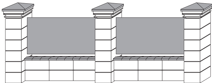
Słupek + poddasze grube + daszek koperta, podmurówka z daszkiem dwuspadowym
